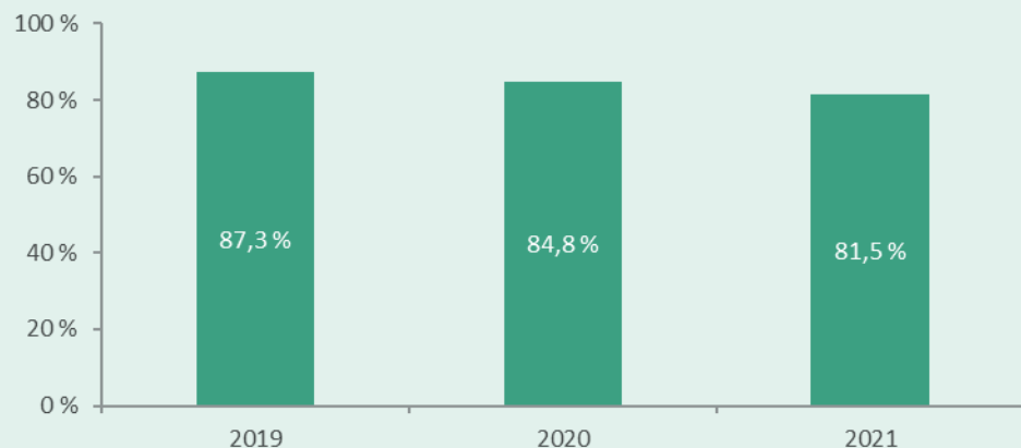
Kombinirani količnik
