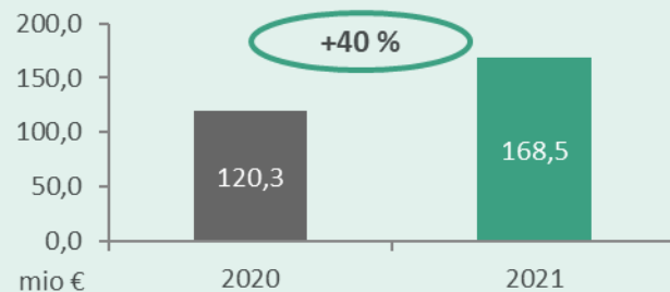
Kosmate premije
