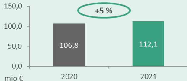
Kosmate premije
