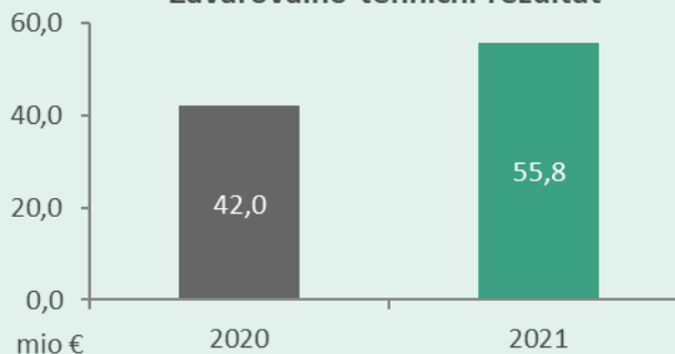
Zavarovalno-tehnični rezultat
