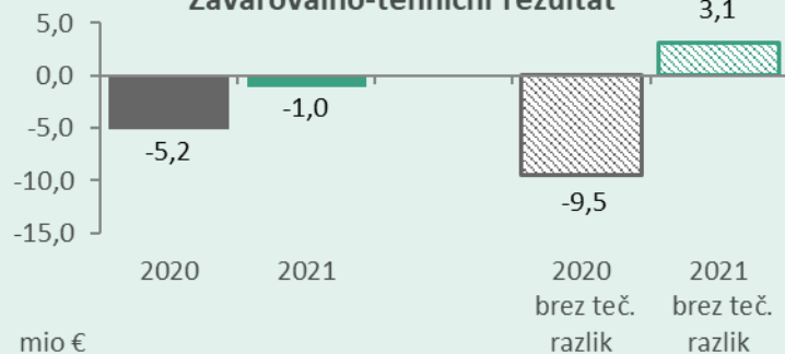
Zavarovalno-tehnični rezultat
