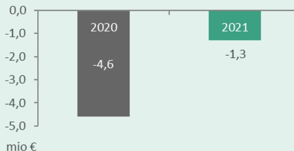
Zavarovalno-tehnični rezultat
