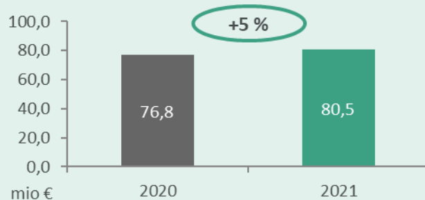
Kosmate premije
