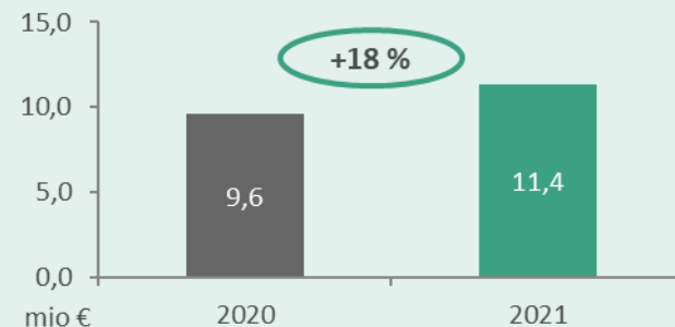
Obratovalni stroški
