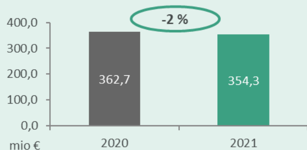
Kosmate premije
