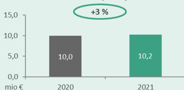
Kosmate premije
