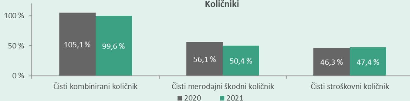
Količniki
